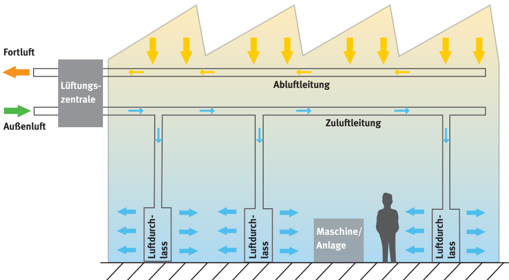
Abb. 7: Prinzip der Schichtlüftung
