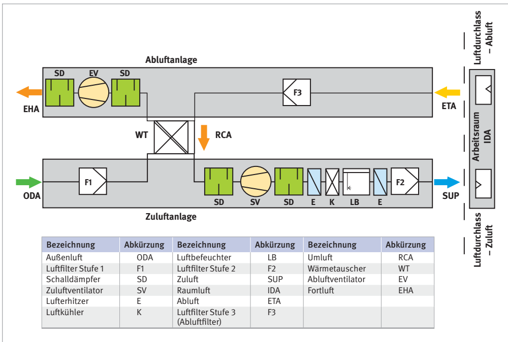
Abb. 5: Schematischer Aufbau einer RLT-Anlage
