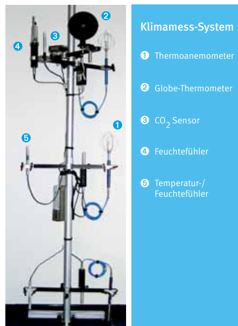
Abb. 3: Klimamess-System mit verschiedenen Sensoren
